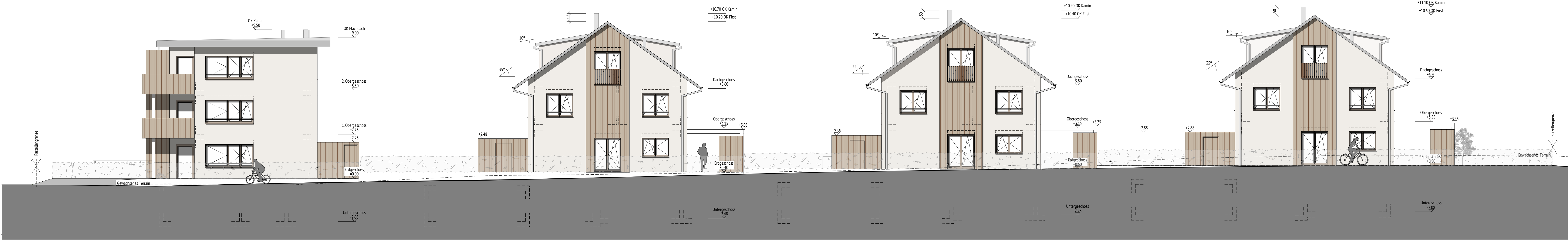
Südfassaden Wiesenstrasse
